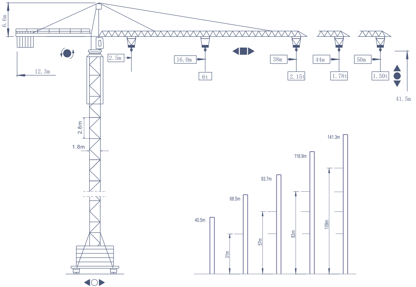
底座固定式 Chassis stationary
